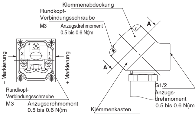
Ansicht A-A
