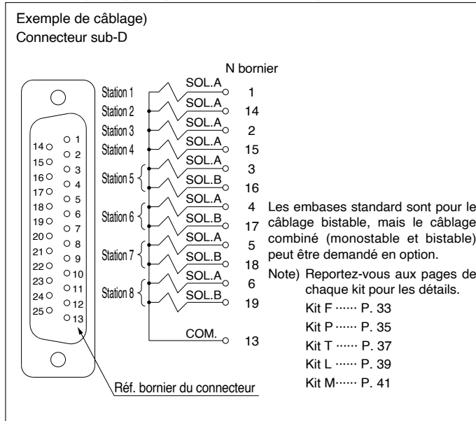
Caractéristiques spécifiques du câblage électrique [-K]
