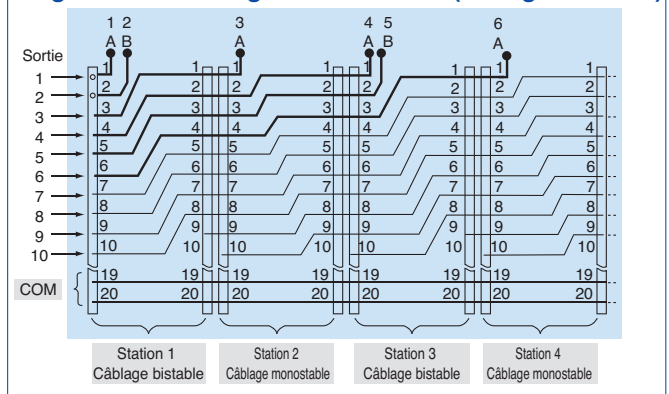
Diagramme de câblage de connecteur (câblage combiné)
