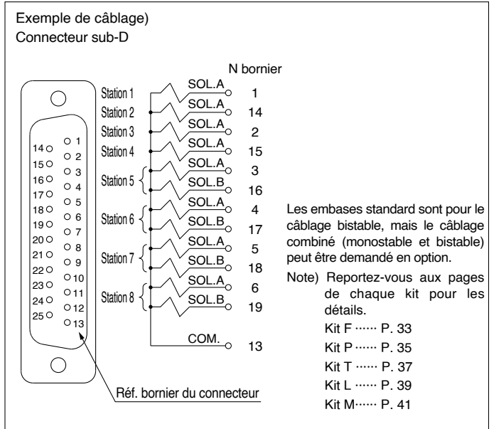
Caractéristiques spécifiques du câblage électrique [-K]
