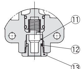
Coupe d'orifice d'échappement
