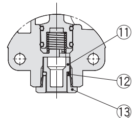
Coupe de l'échappement
