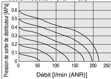
Pression réduite A1 (P R →A), Pression réduite B1 (P R →B)
