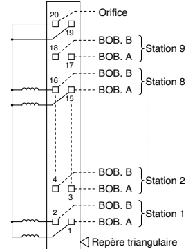
Câble plat 10PG/16PG (20 broches)
