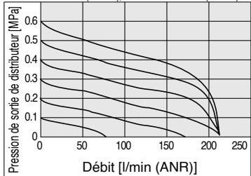
SV3000 Pression réduite P (P R →A,B)
