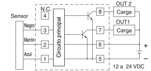
PF2D300-A(-M)
