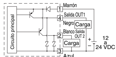
PF2W704T-67(-M)
