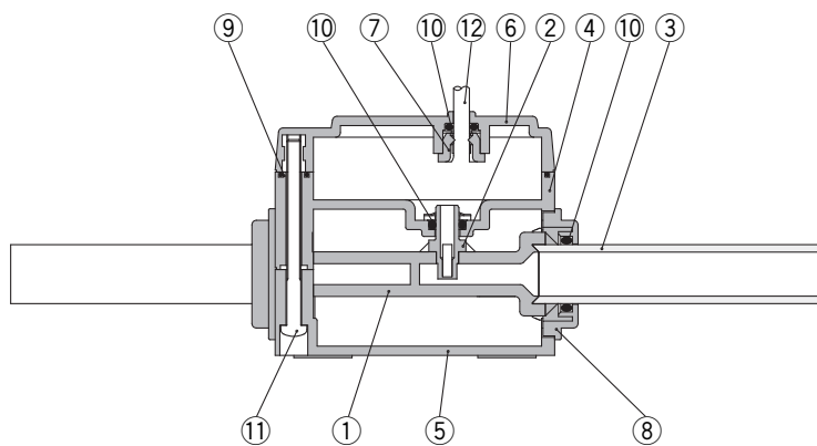
PF2D504/520
