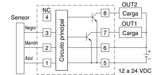
PF2A3□0-A
