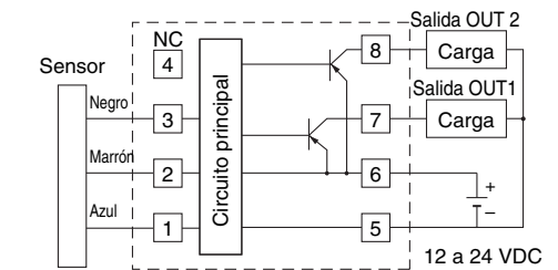
PF2A3□1-A
