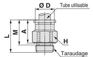
Dimensions de la collerette de déblocage
