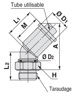
Dimensions de la colerette de déblocage
