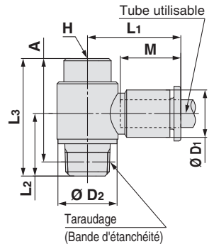
Dimensions de la colerette de déblocage
