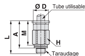
Dimensions de la collerette de déblocage
