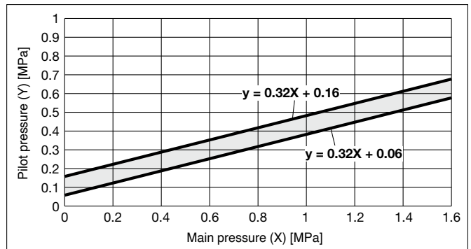
JSB64-ST40A□-5S
