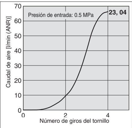
JASV-LE□□-M3 OUT-EXH. Caudal
