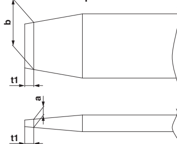
Forma de la punta del destornillador
