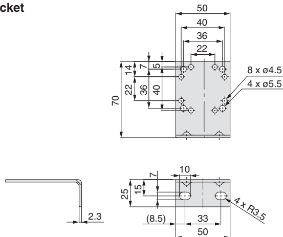
L-bracket
