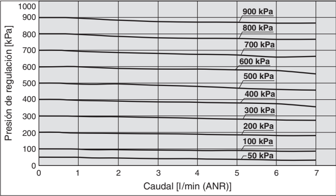
Características de caudal
