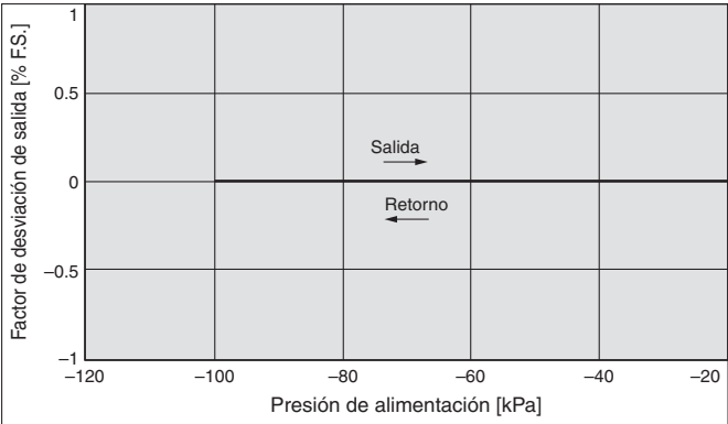
Características de presión Presión de regulación: -10 kPa
