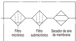
IDG60 a 100M2 IDG60H a 100HM2
