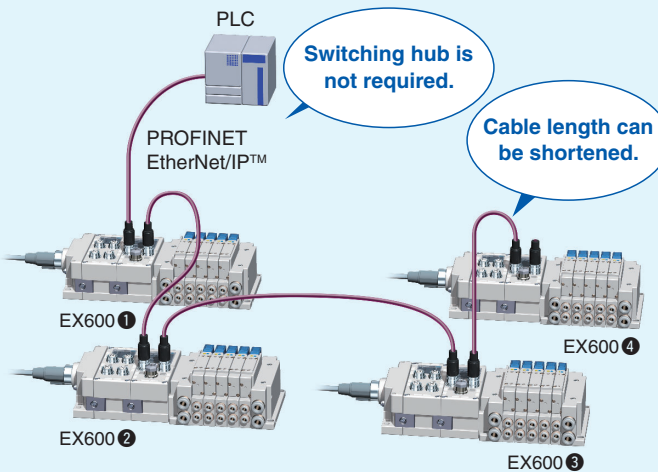
Linear type
