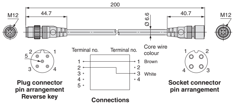
EX9-AC002-4
