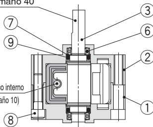
Modelo de eje simple
