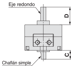
Eje doble/CDRB2□J
