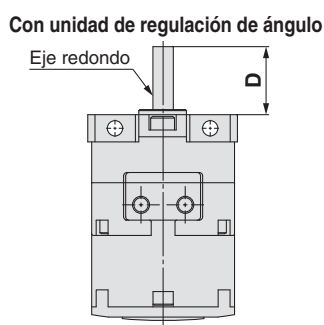
Eje doble/CRBU2JU
