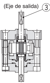
Modelo de eje doble
