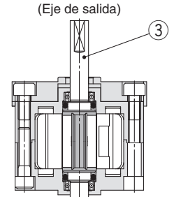
Modelo de eje doble
