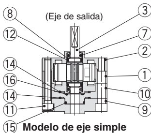
Modelo de eje simple
