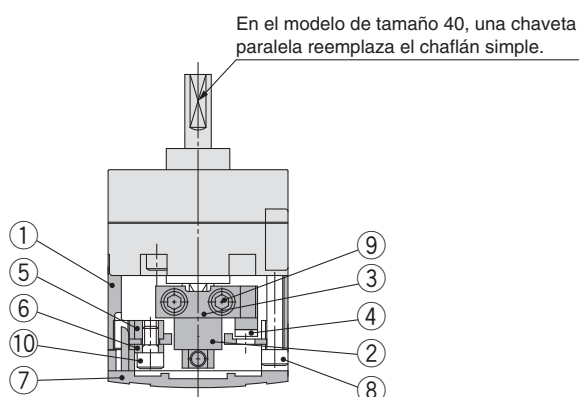
Paleta simple
