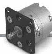
Conjunto de brida para C□RB2F□□15 Ref.: P211090-2
