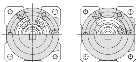
Paleta simple
