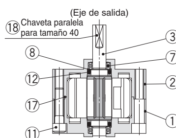
Modelo de eje simple
