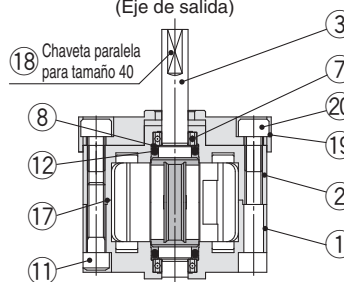
Modelo de eje simple
