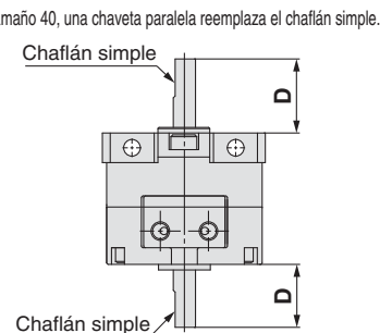
Eje simple/CRBU2Y
