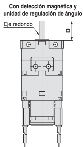
Eje doble/CRBU2JU
