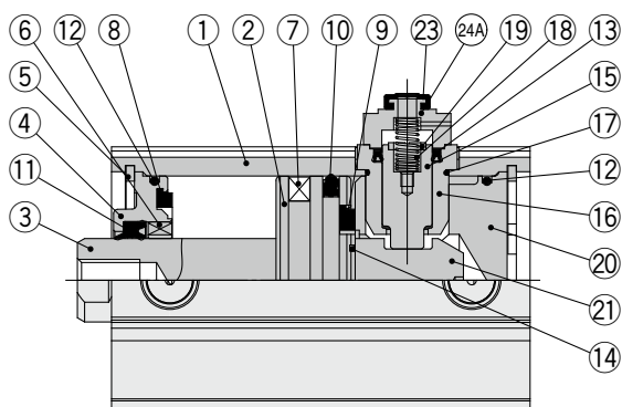
Verrouillage arrière
