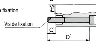
Montage fond avant
