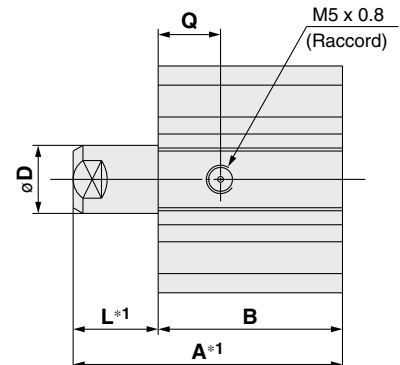
Tige sortie
