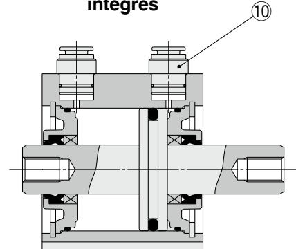
Raccords instantanés intégrés
