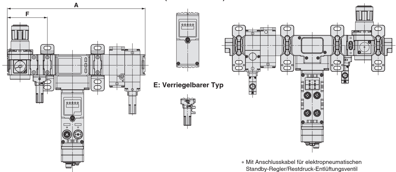
AMS20/30/40/60B-H00D (Ohne Anbauteile)
