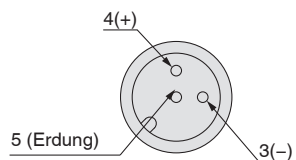
Detailansicht: M12 a-kodierter Anschluss
