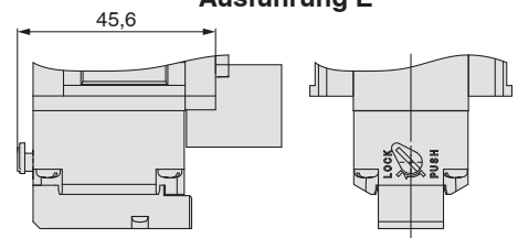
Detailansicht: Handhilfsbetätigung (für manuelle Betätigung) Ausführung E
