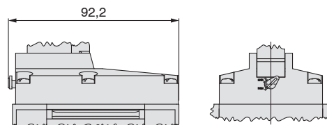
Detailansicht: Handhilfsbetätigung (für manuelle Betätigung) Ausführung E
