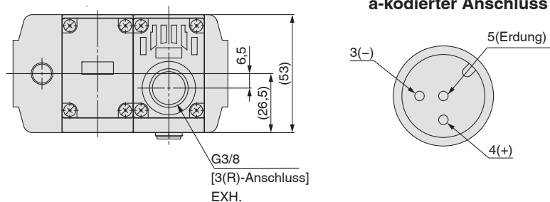
Detailansicht: M12 a-kodierter Anschluss
