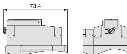
Detailansicht: Handhilfsbetätigung (für manuelle Betätigung)
