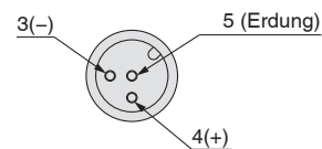
Detailansicht: M12 a-kodierter Anschluss
