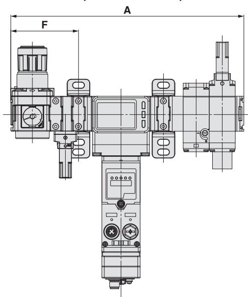
AMS20/30/40/60B-H00C (Ohne Anbauteile)
