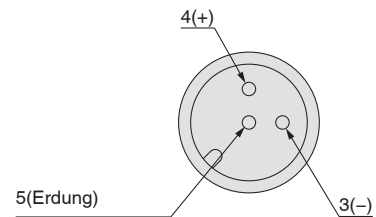
Detailansicht: M12 b-kodierter Anschluss
