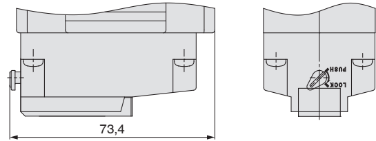
Detailansicht: Handhilfsbetätigung (für manuelle Betätigung)
