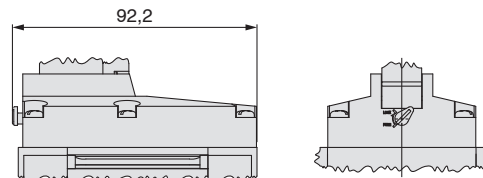
Detailansicht: Handhilfsbetätigung (für manuelle Betätigung) Ausführung E
