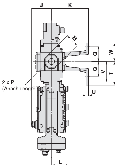
AMS20/30/40/60B-H00C (Ohne Anbauteile)
