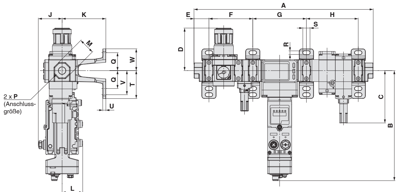
AMS20/30/40/60B-H00D (Ohne Anbauteile)
