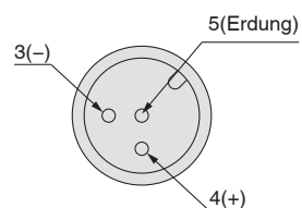
Detailansicht: M12 a-kodierter Anschluss
