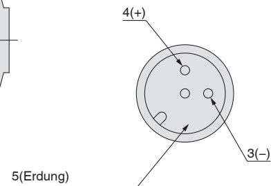
Detailansicht: M12 b-kodierter Anschluss
