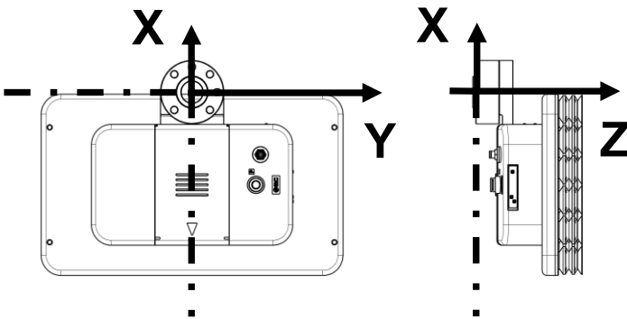
Fig 6. Offset flange + Flange Y
