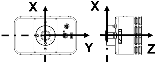
Fig 16. Straight flange
