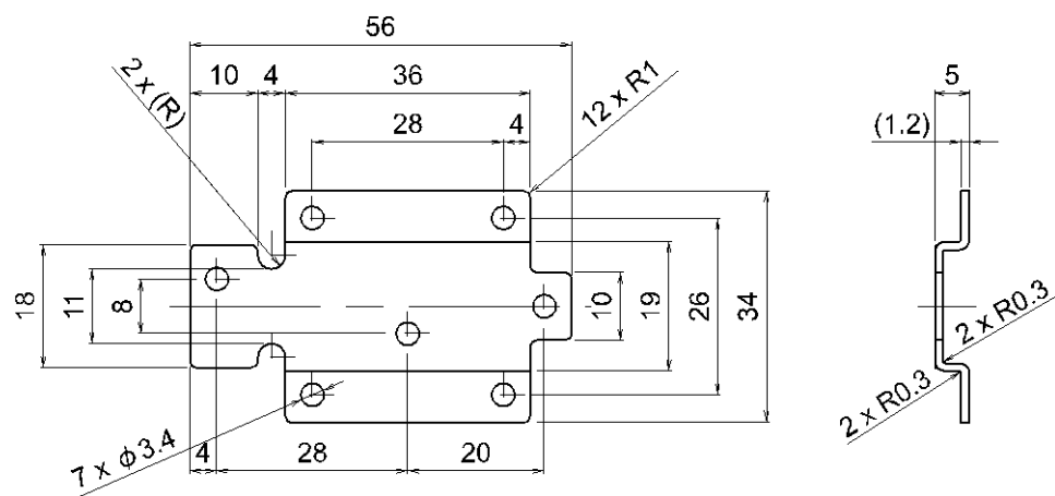
Bracket (ZS-33-MS)
