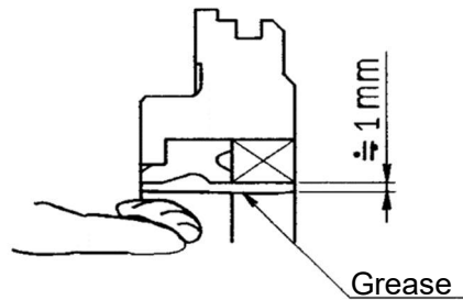
Fig. 10 Rod seal
