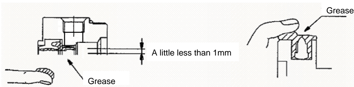
Fig. 6 Rod seal
