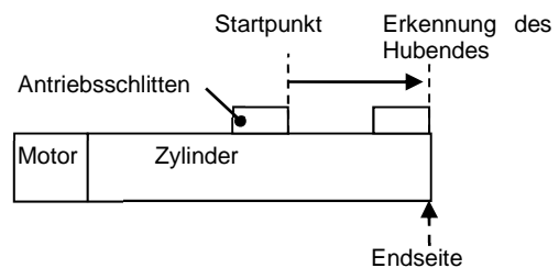
Befehl der Referenzfahrt in Richtung Endseite
