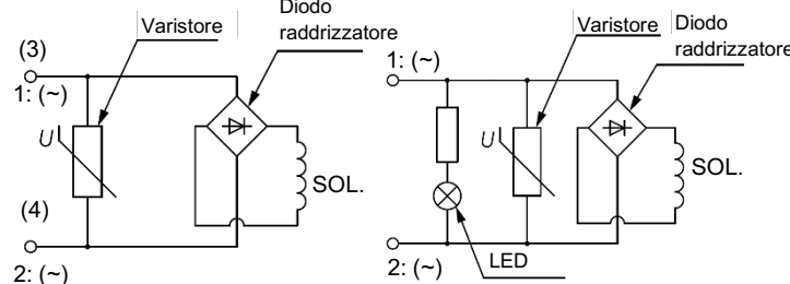
Figura 11. Grommet / terminale DIN / condotto con circuito di protezione / connettore M12 (3,4)
