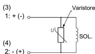
Figura 9. Grommet / terminale DIN / condotto con soppressore di sovratensione / connettore M12 (3,4)
