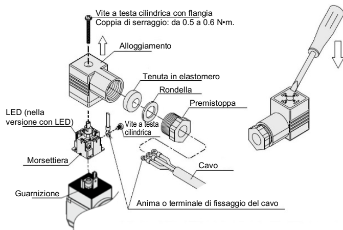
Figura 5. Costruzione del connettore DIN JSX20/30
