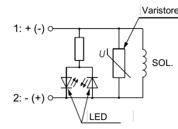
Figura 10. Terminale DIN con LED e circuito di protezione
