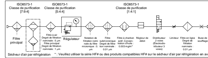
Circuit d'équipement pneumatique d'une soufflerie d'air pour une application alimentaire (exemple)
