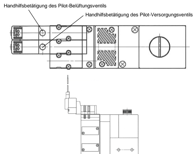
Kombination aus Versorgungs- und Belüftungsventil: K2
