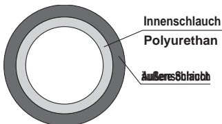
doppellagiger Polyurethan-Schlauch, schwer entflammbar (Schnitt)
