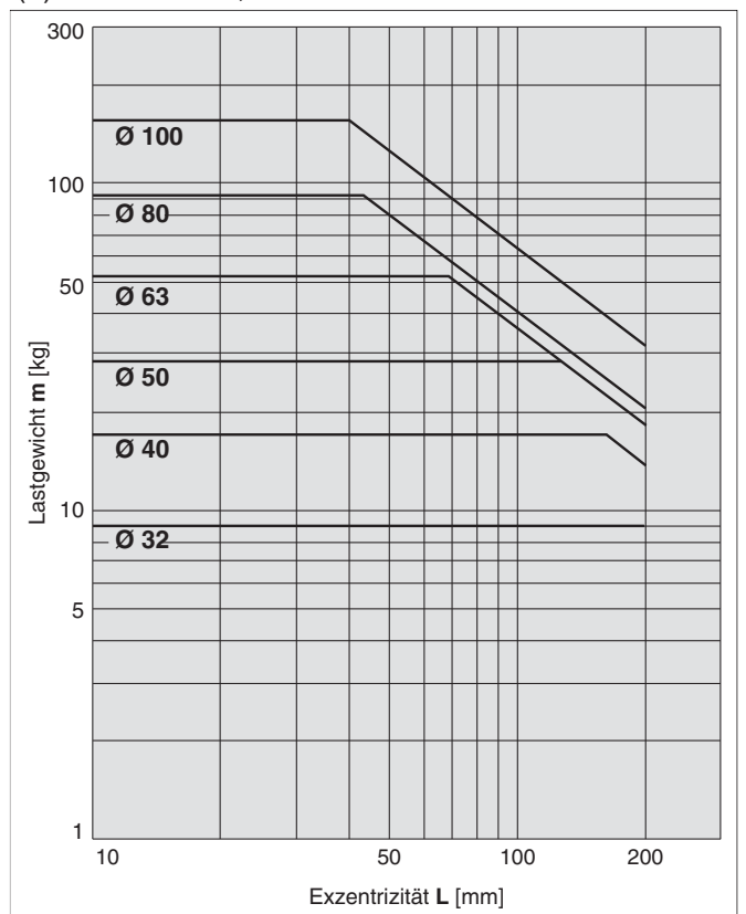
(8) Über Hub 50, V = max. 200 mm/s
